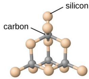
silicon carbide
